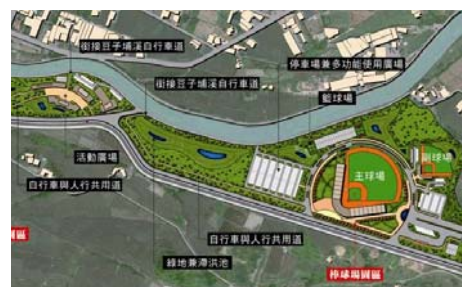
大新竹風光計畫配置示意圖
